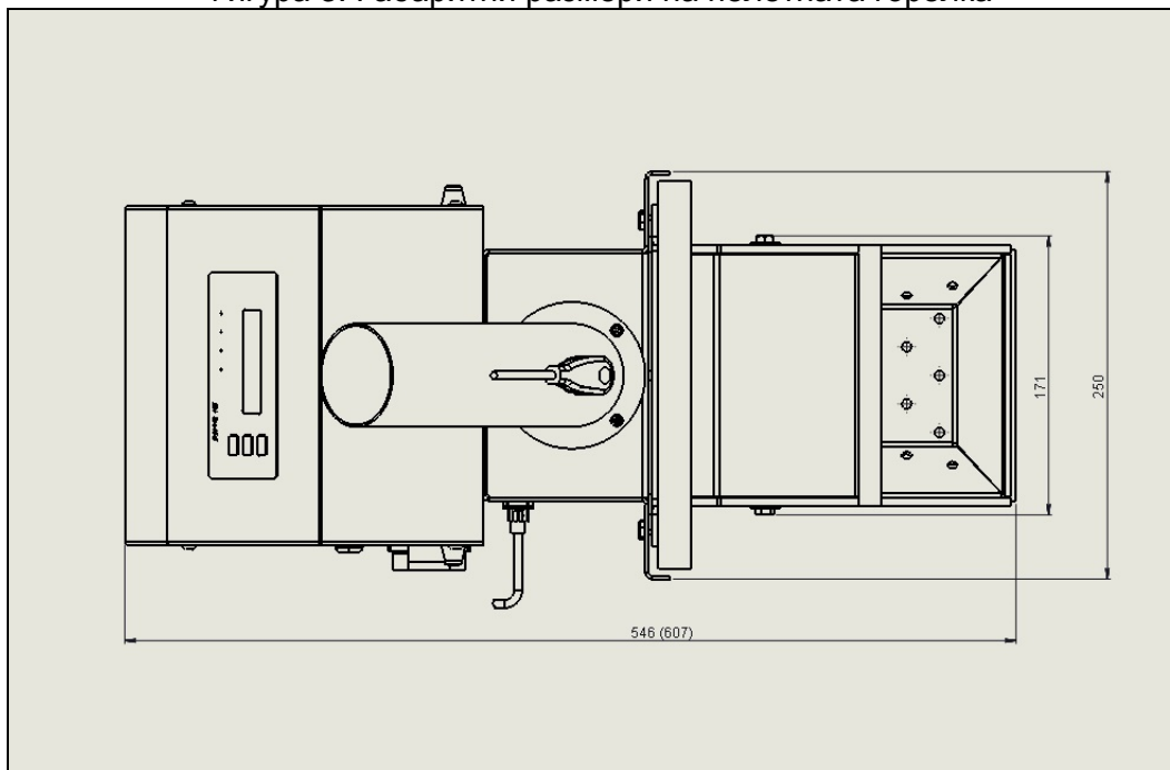
Фигура 3. Габаритни размери на пелетната горелка
