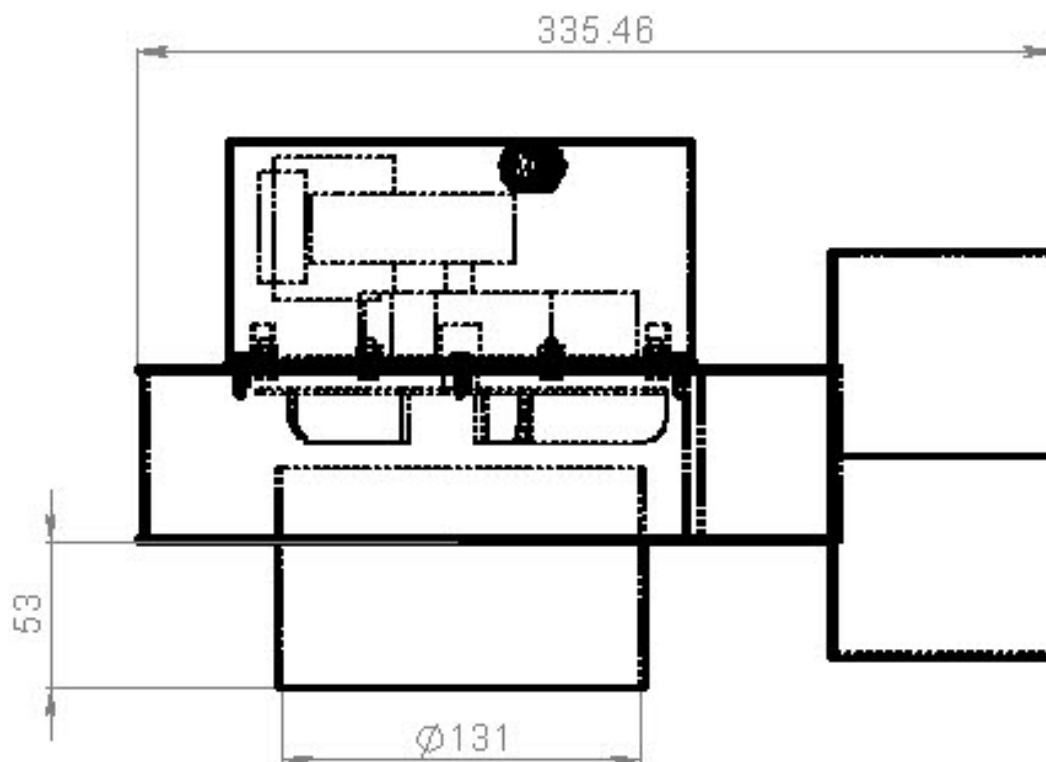
Фигура 2.2. Информация за габаритните и присъединителните размери на вентилаторната група – поглед отгоре ;
