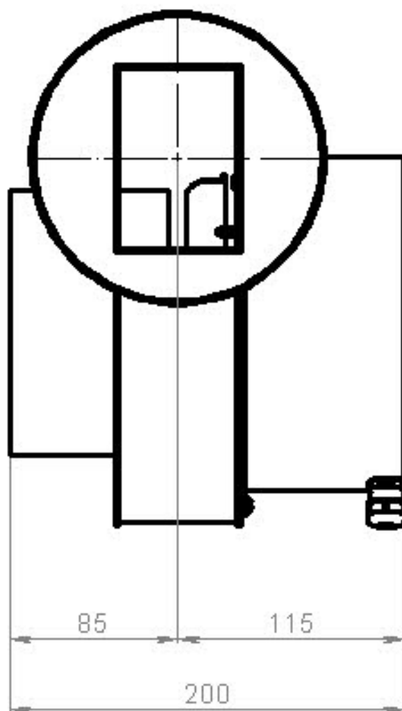
Фигура 2.3. Информация за габаритните и присъединителните размери на вентилаторната група – поглед откъм изходящото сечение на модула;
