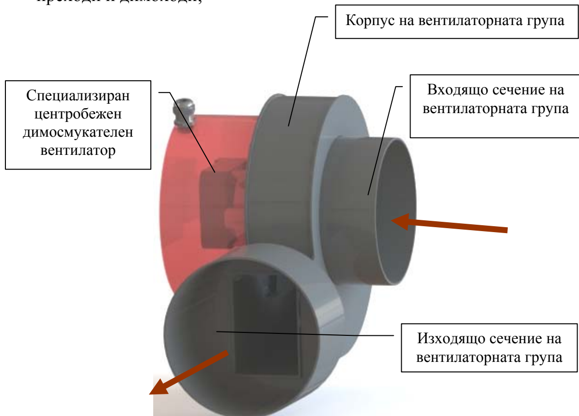
Фигура 3.1. Основни елементи на вентилаторната група за принудително отвеждане на димни газове.
