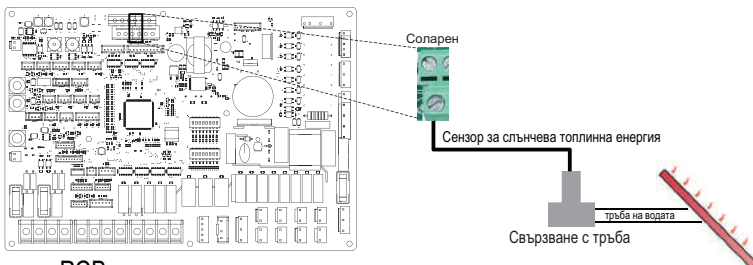
PCB на вътрешно тяло
