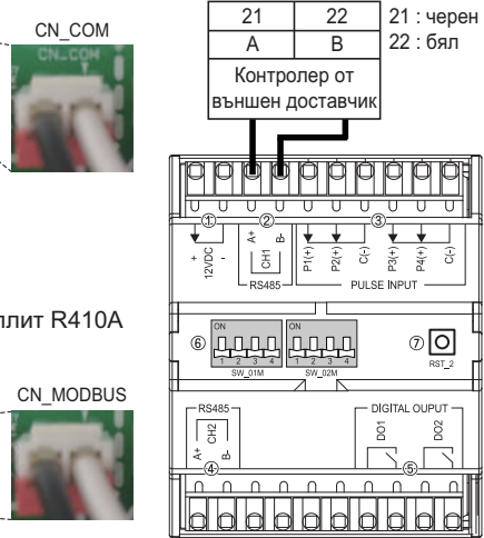
Интерфейс към измервателен уред
