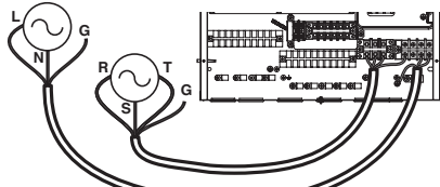
3Ø резервен нагревател (за сплит R410A вътрешно тяло 3 серия)
